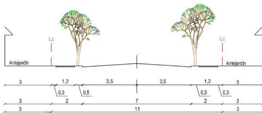
Perfil tipo Calles Corte A-A
