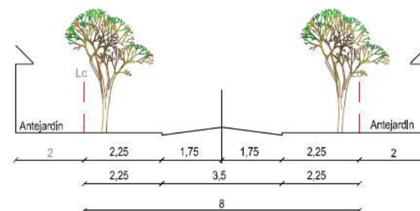
Perfil tipo Pasaje Corte B-B
