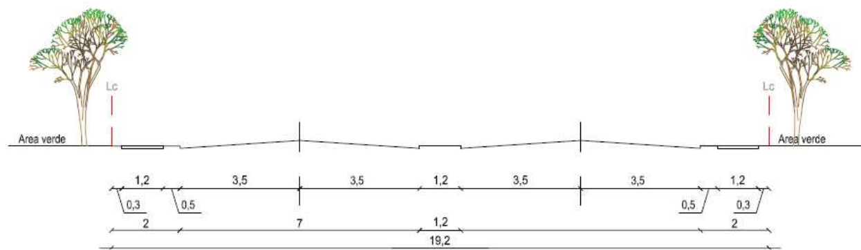
Perfil Acceso Corte C-C
